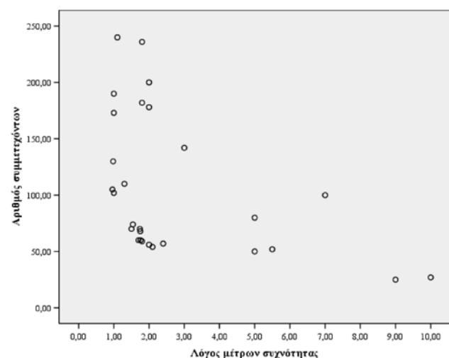
Εικόνα 2. Διάγραμμα «χωνί», με την ύπαρξη ασυμμετρίας να υποδηλώνει την παρουσία σφάλματος δημοσίευσης.
