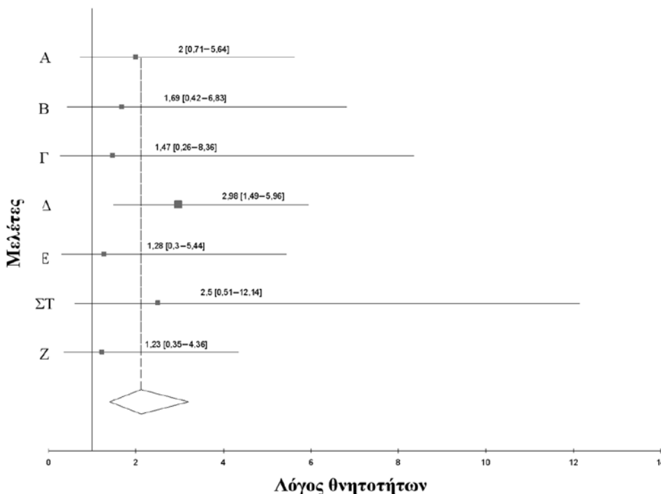
Εικόνα 5. Διάγραμμα «δάσος» που αντιστοιχεί στα αποτελέσματα της μετα-ανάλυσης των 7 κλινικών δοκιμών του πίνακα 1.
